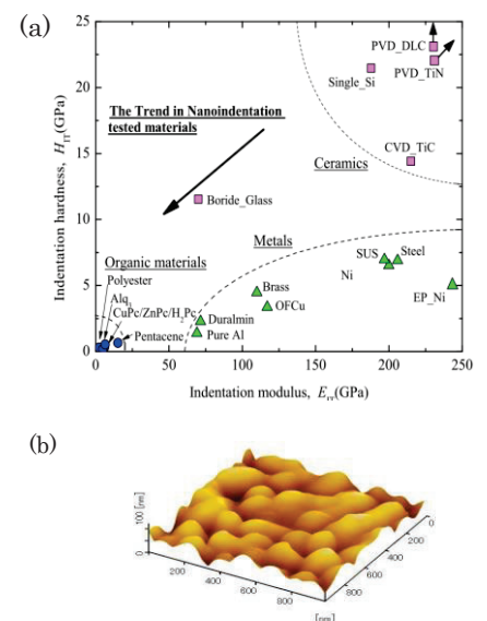
図1 (a)押込み試験に供される材料の変化と(b)ペンタセン有機半導体のSPM像
