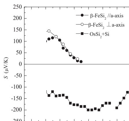
3 シリサイド結晶のゼーベック係数の温度依存性
