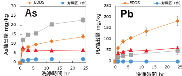
ヒ素(左), 鉛(右)汚染土壌のキレート洗浄
