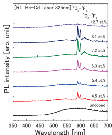
図 1 Eu 添加 \text{SnO}_2 の発光スペクトルの濃度依存性
