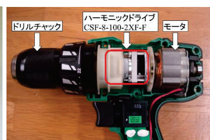
電動ドライバの改良
